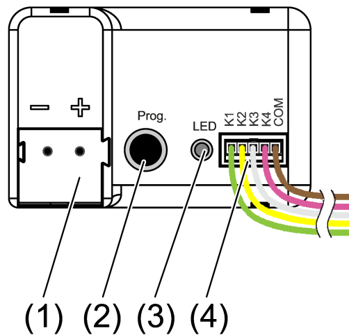
Bild 2: Gerätevariante 4fach
