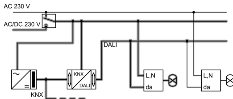
Figura 4: Lámparas de emergencia, instalación KNX y pasarela DALI alimentadas mediante suministro central de seguridad
