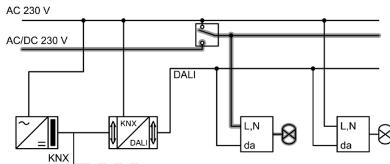
Figura 3: Lámparas de emergencia alimentadas mediante suministro central de seguridad
