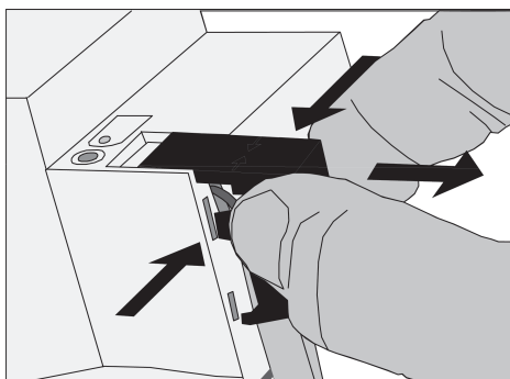
rysunek 5: Zdjęcie klapy pokrywy
