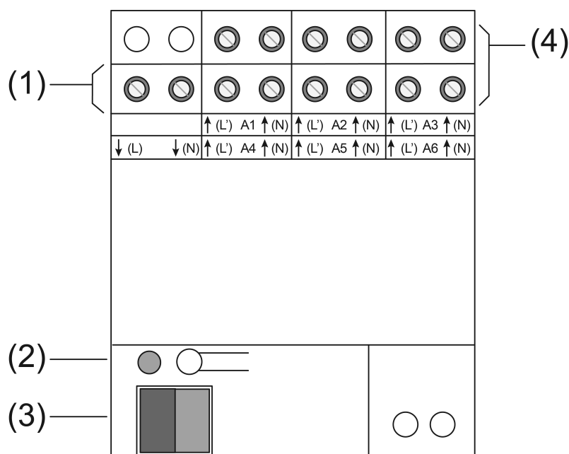
rysunek 1: Widok z przodu
