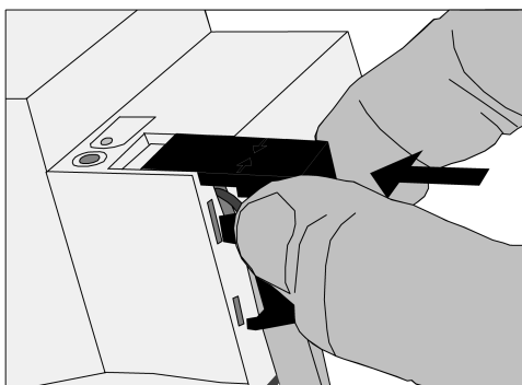
rysunek 4: Nałożenie klapy pokrywy
