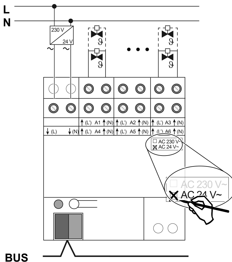
rysunek 3: Podłączenie napędów nastawczych 24 V
