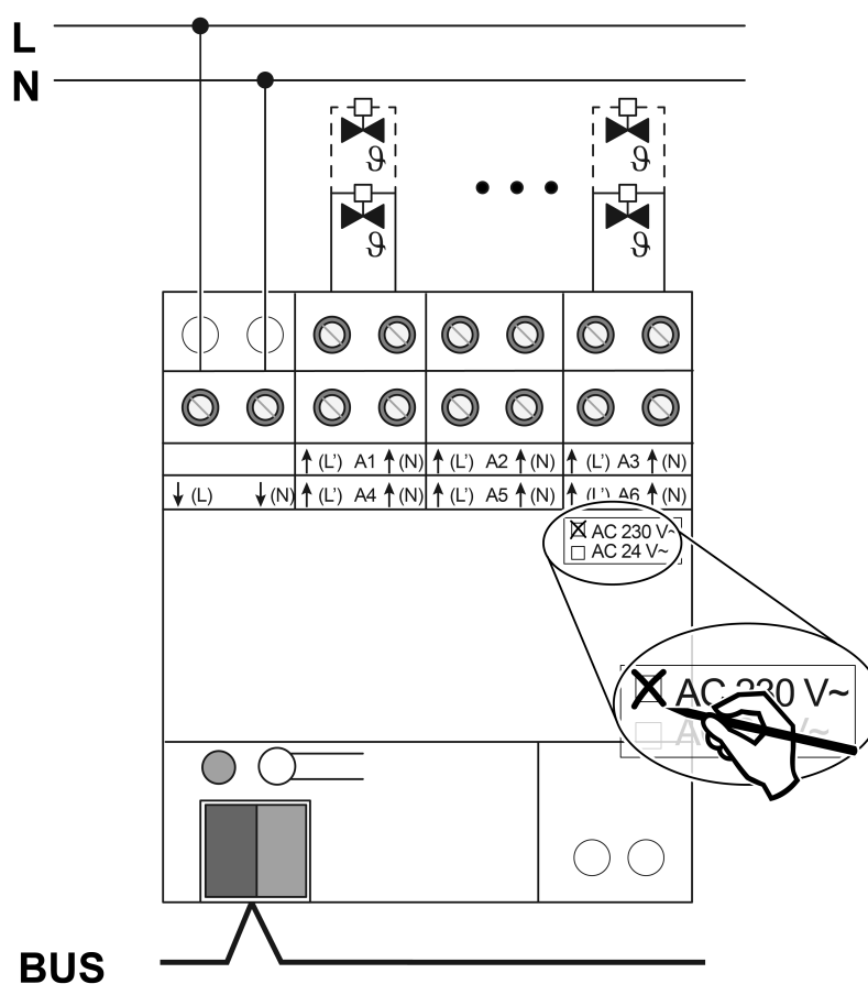
rysunek 2: Podłączenie napędów nastawczych 230 V
